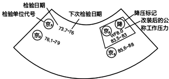
图 8-3 气瓶的检验钢印标记
