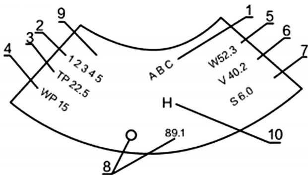
图 8-2 气瓶的制造钢印标记
